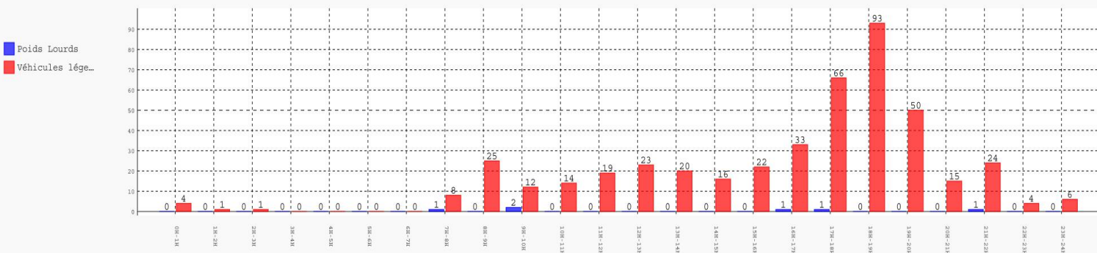
Horaires de passage en tranche 60-70 Km/h Sens1 (id SIG :19026)
