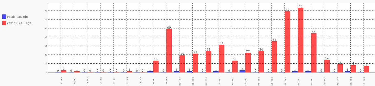
Horaires de passage en tranche 50-60 Km/h Sens1 (id SIG :19026)
